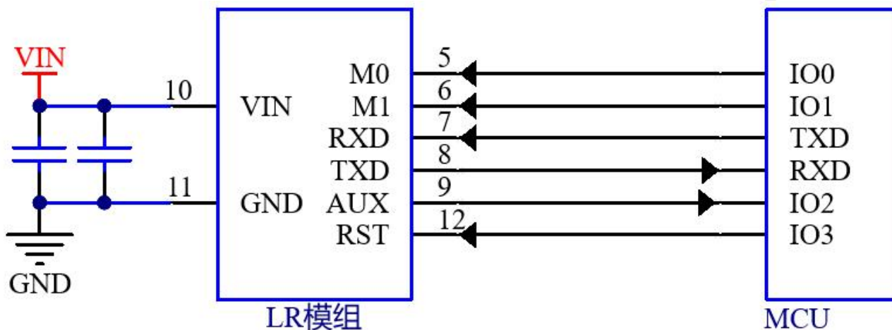
图 2：模块最小系统图
