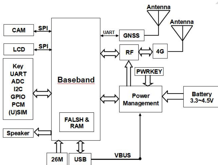
图 1：功能框图
