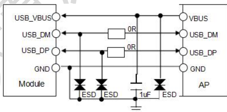
图 11: (U)SIM 卡信号连接电路
