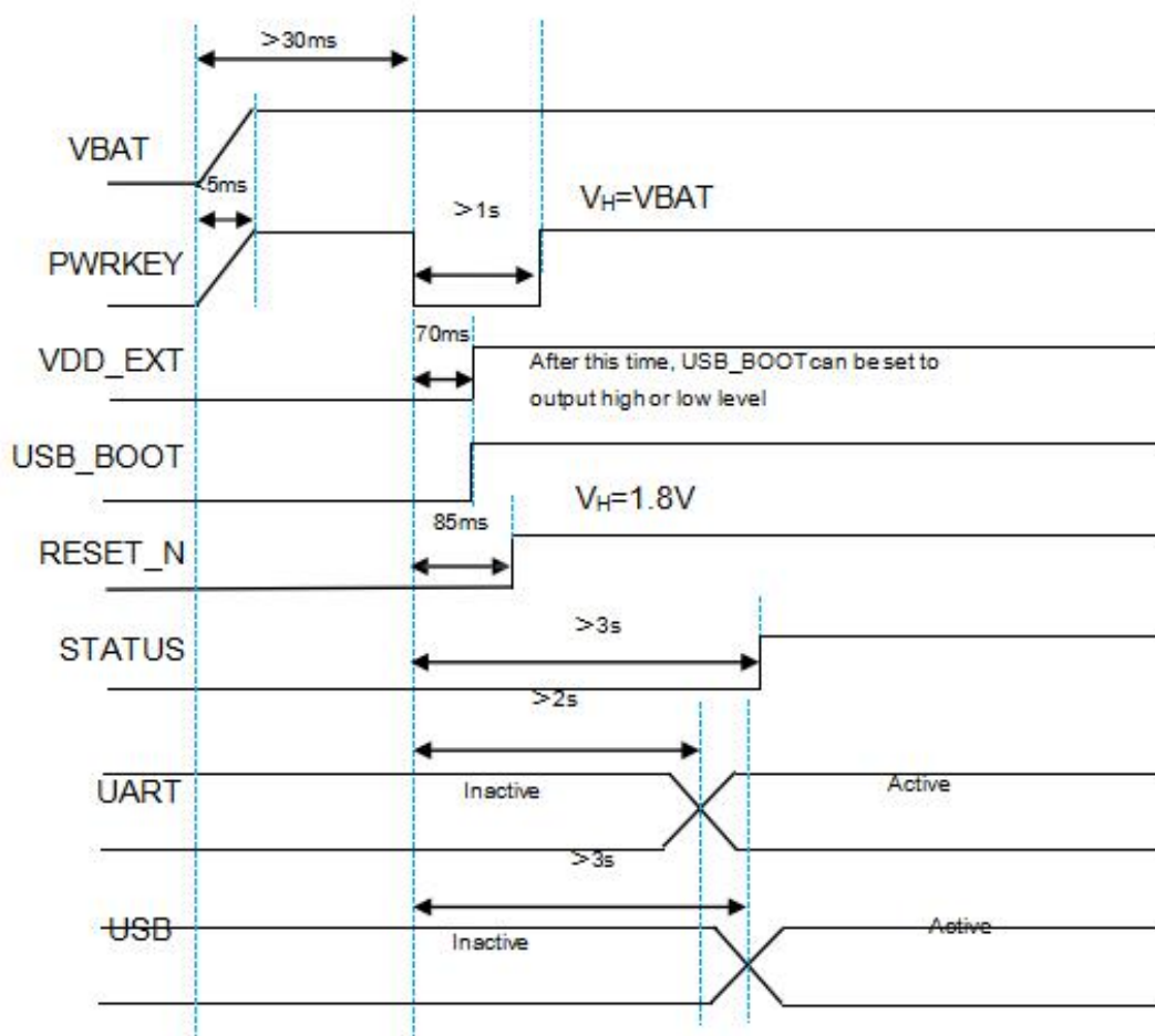
图 16: 上电时序图
