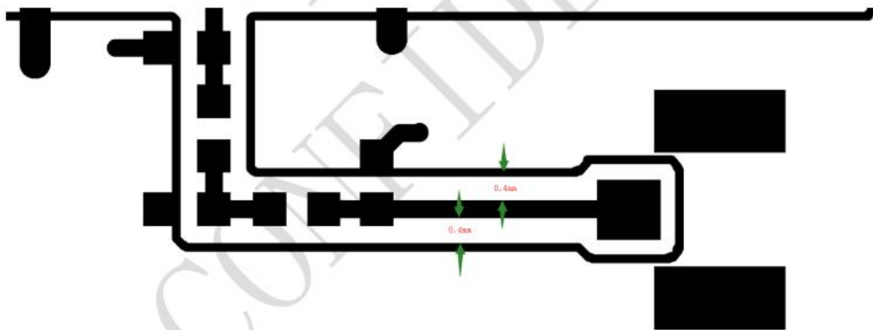
图 18：天线路径参考设计
