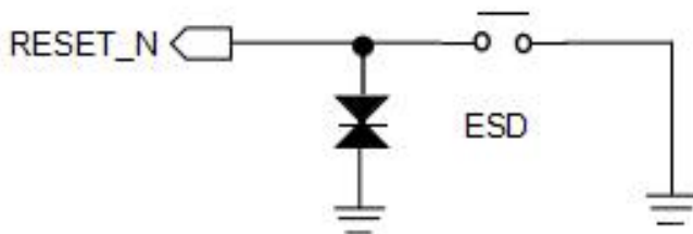
图 9：复位参考电路
