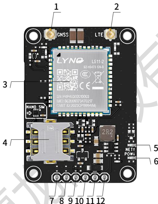
图 3: CT511-A/CT511N-A 底板定义
