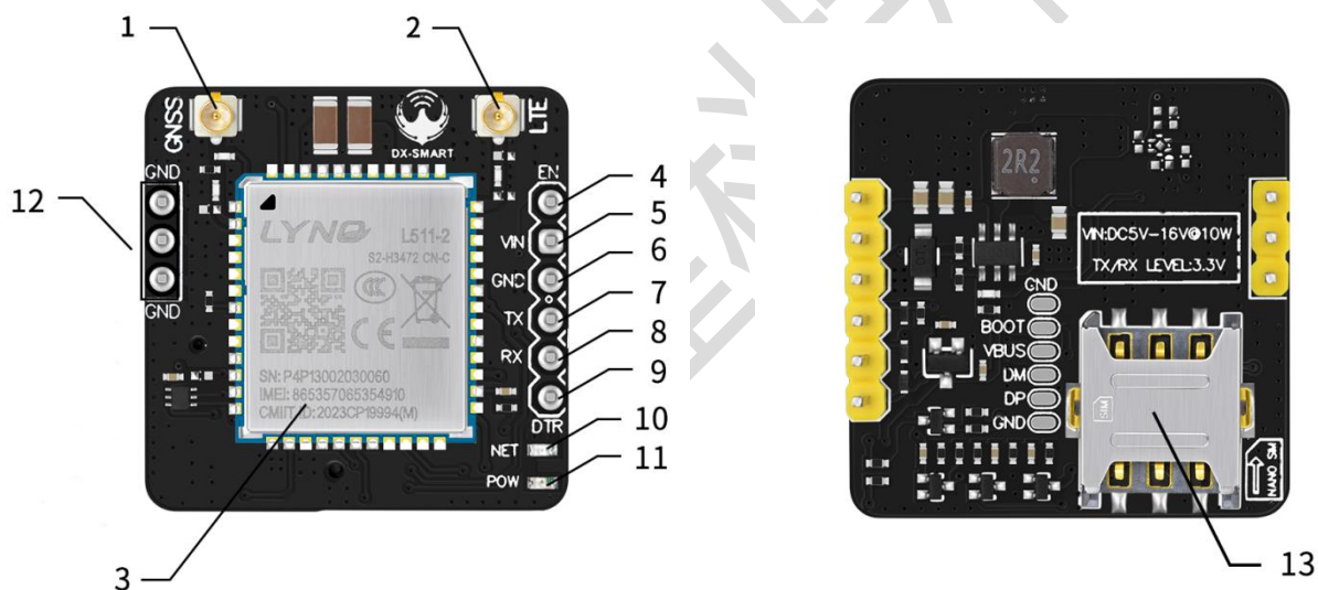
图 4：CT511-B/CT511N-Bmini 底板定义
