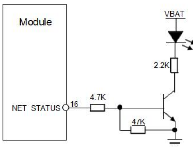
图 15: NET_STATUS 电路
