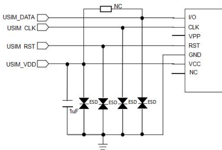
图 10: (U)SIM 卡信号连接电路
