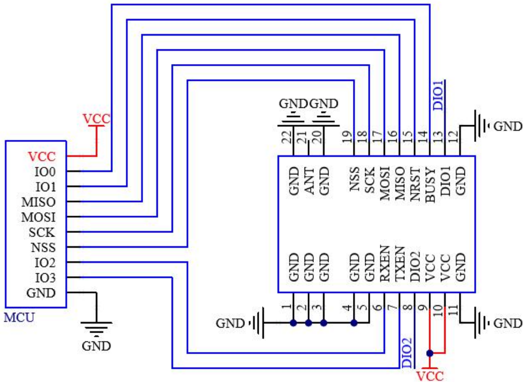
图 3：基本电路
