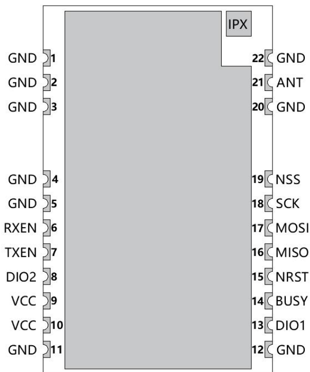
图 1：模块引脚定义
