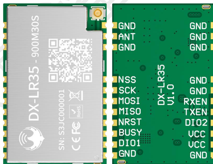
图 6：模块俯视图和底视图
