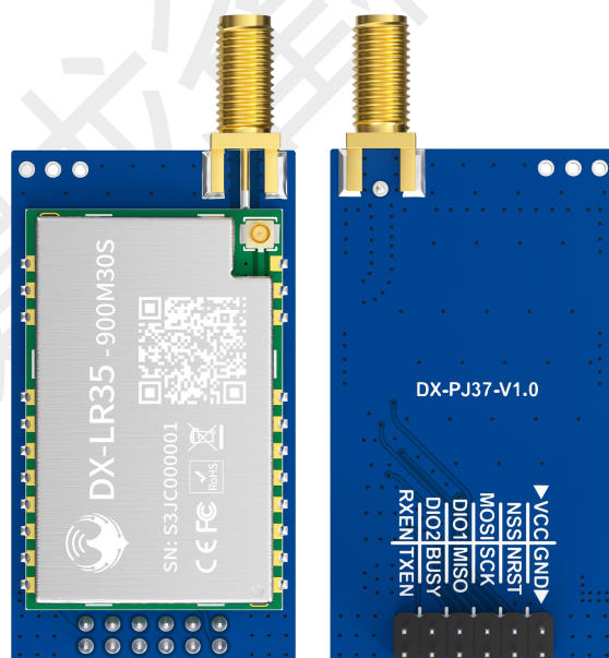
图 8：底板俯视图和底视图
