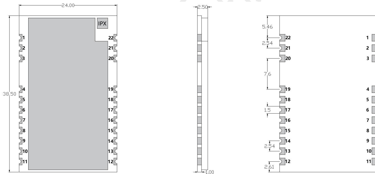
图 4：模块俯视，侧视及底视尺寸图
