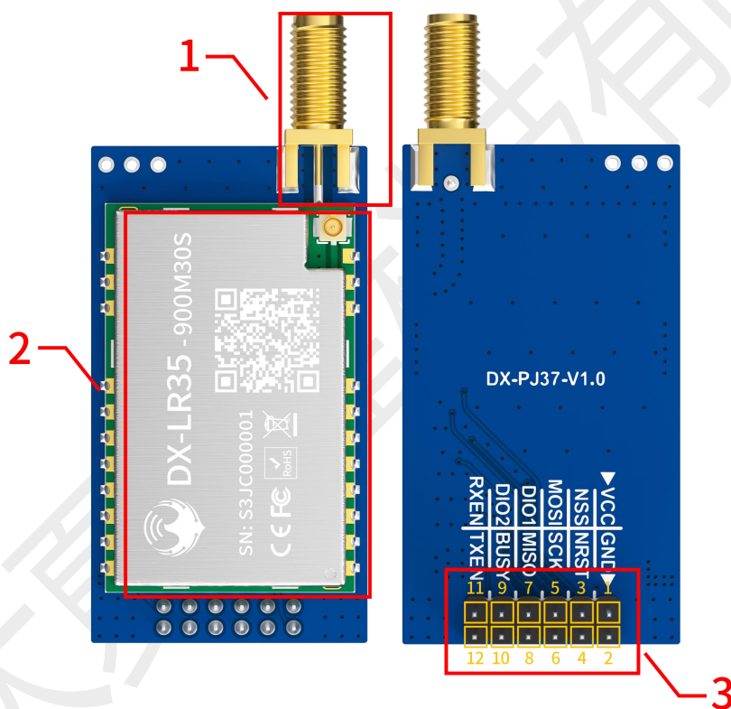
图 2：底板版块定义
