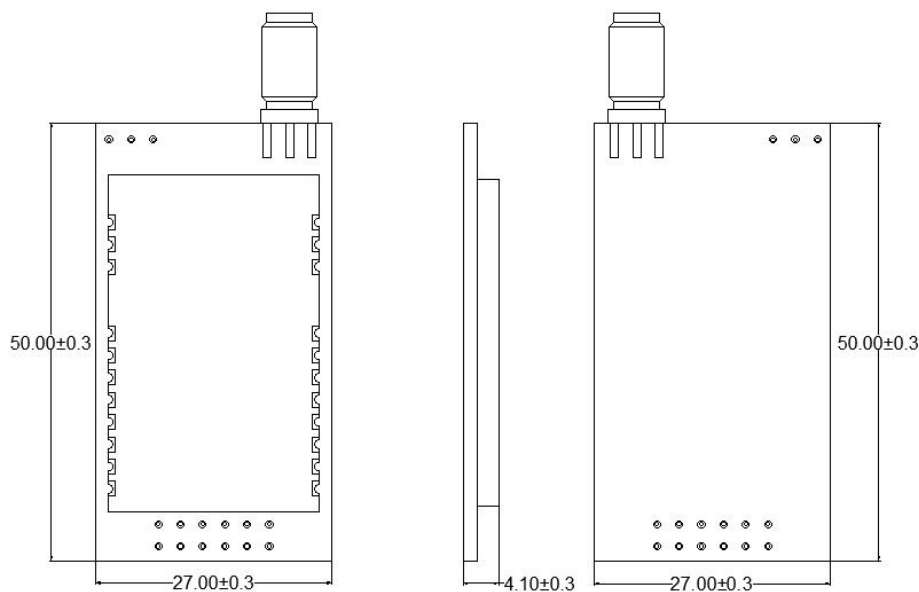
图 7：底板俯视，侧视及底视尺寸图
