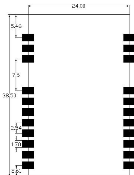
图 5：建议封装尺寸底视图
