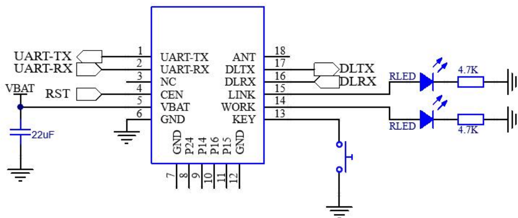
图 14: 典型应用电路
