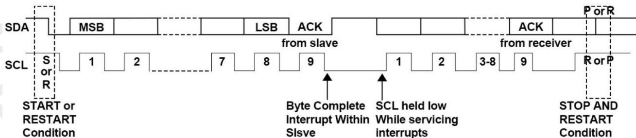
图 9: I2C 通信时序图
