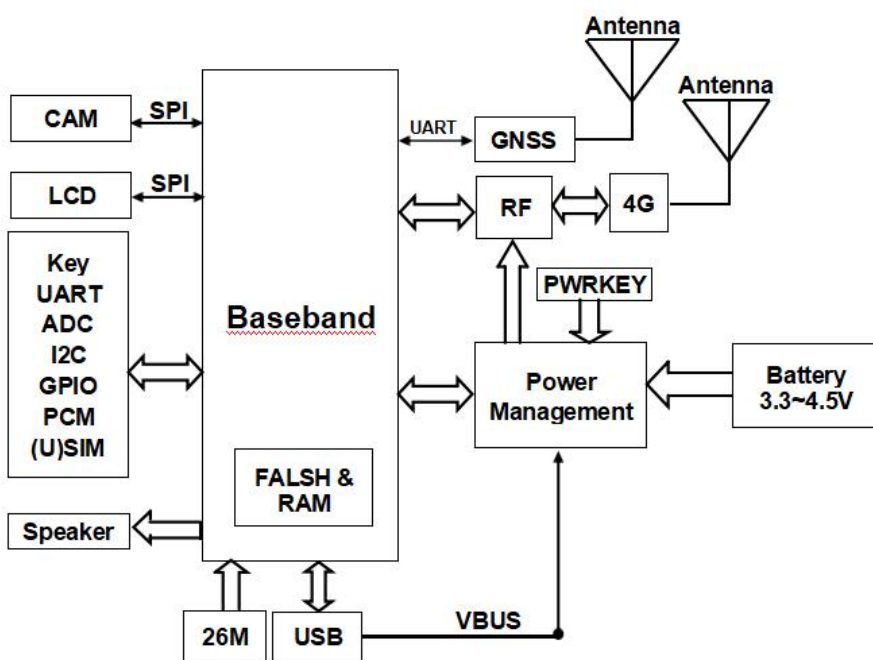
图 1：功能框图
