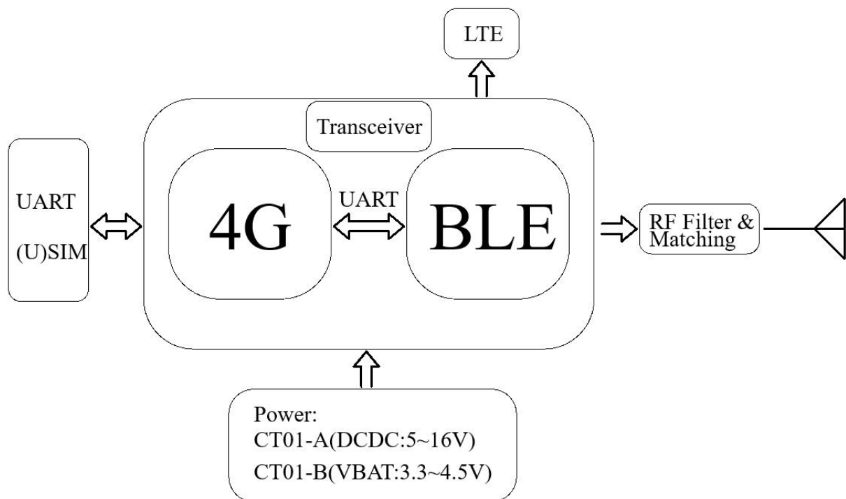
图 1：功能框图
