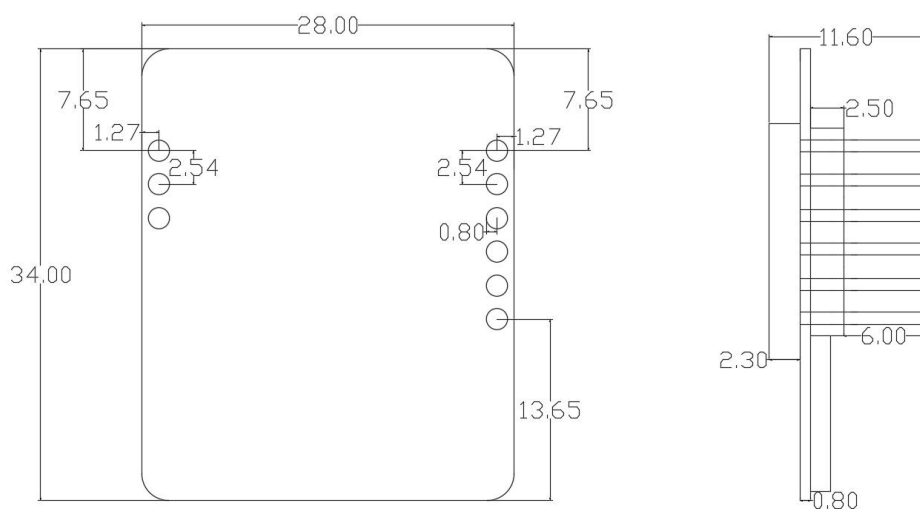
图 6: 模块尺寸
