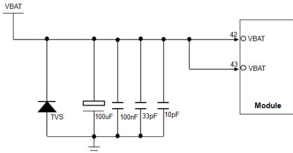
图 4：电池供电参考电路( CT01-B 模块 )
