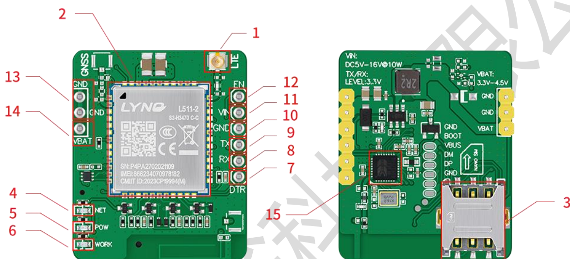
图 2：底板定义
