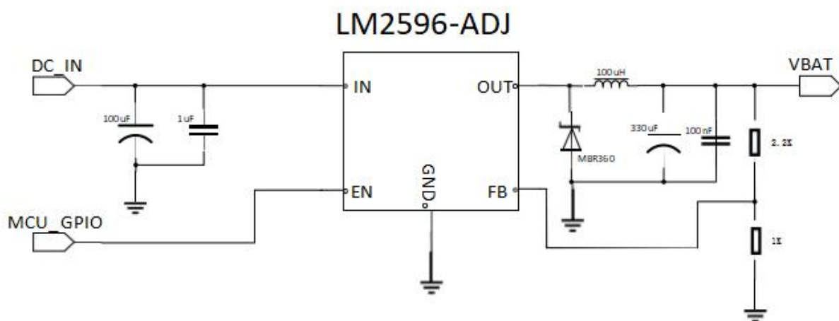
图 3：DC/DC 供电参考电路( CT01-A 模块 )
